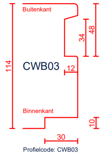
Lekdorpelgroef & vensterbankspanning 10x30
