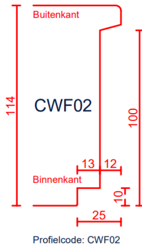
Lekdorpelspanning & vensterbankspanning 10x25
