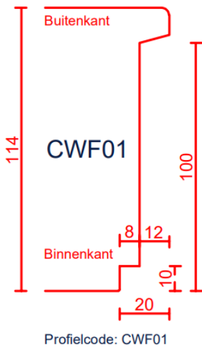
Lekdorpelspanning & vensterbankspanning 10x20
