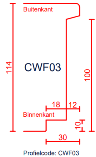
Lekdorpelspanning & vensterbankspanning 10x30
