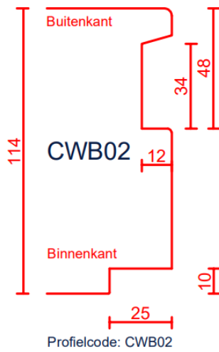
Lekdorpelgroef & vensterbankspanning 10x25
