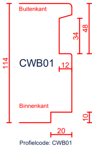
Lekdorpelgroef & vensterbankspanning 10x20
